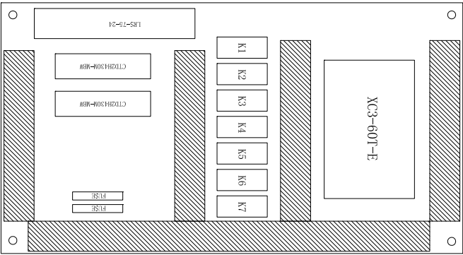
主电盘布局图
