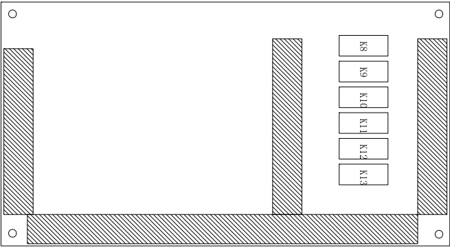
副电盘布局图
